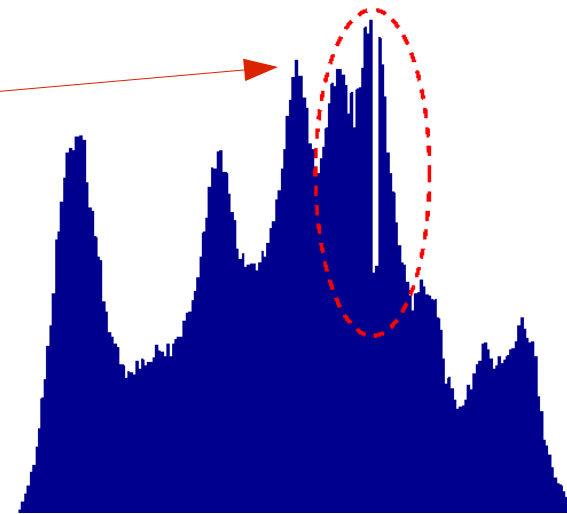
Imagen Ni2003
