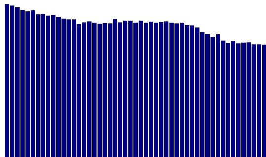
Imagen HSPE
