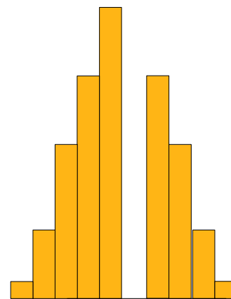
Histograma desplazado
