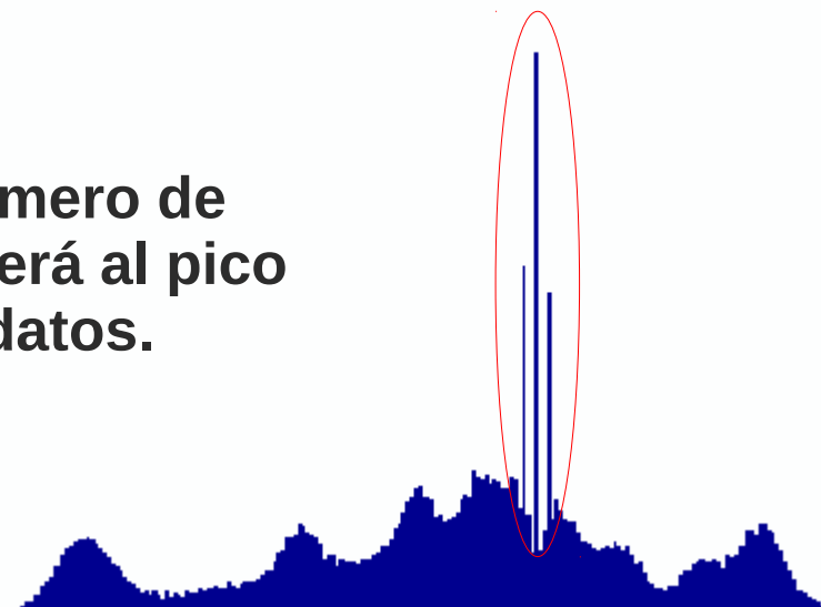
Imagen Mohsenzadeh 2009
